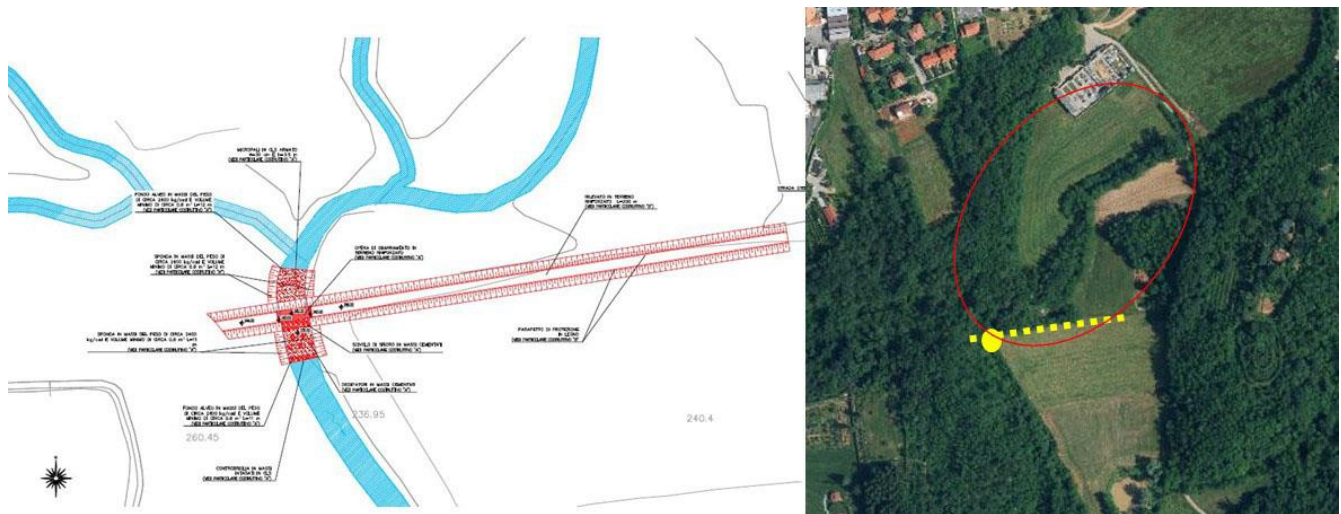
Figura 3: Area di Monte. Stralcio planimetrico dell'opera in oggetto e suo posizionamento entro l'area di intervento.
