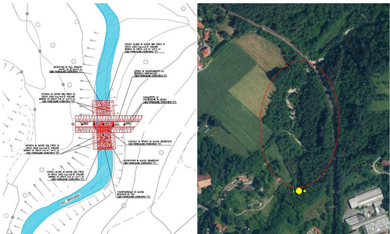
Figura 4: Area di Valle. Stralcio planimetrico dell'opera in oggetto e suo posizionamento entro l'area di intervento.
