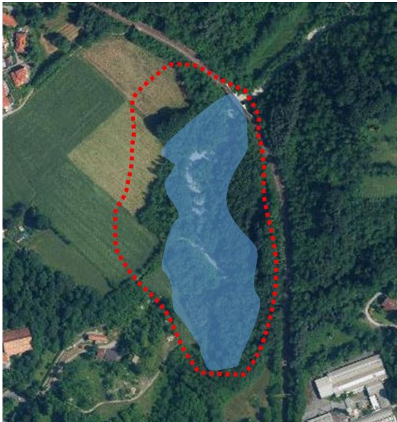
Figura 18: Area di valle. In blu è indicata l'area di esondazione controllata. In rosso l'area di buffer.
