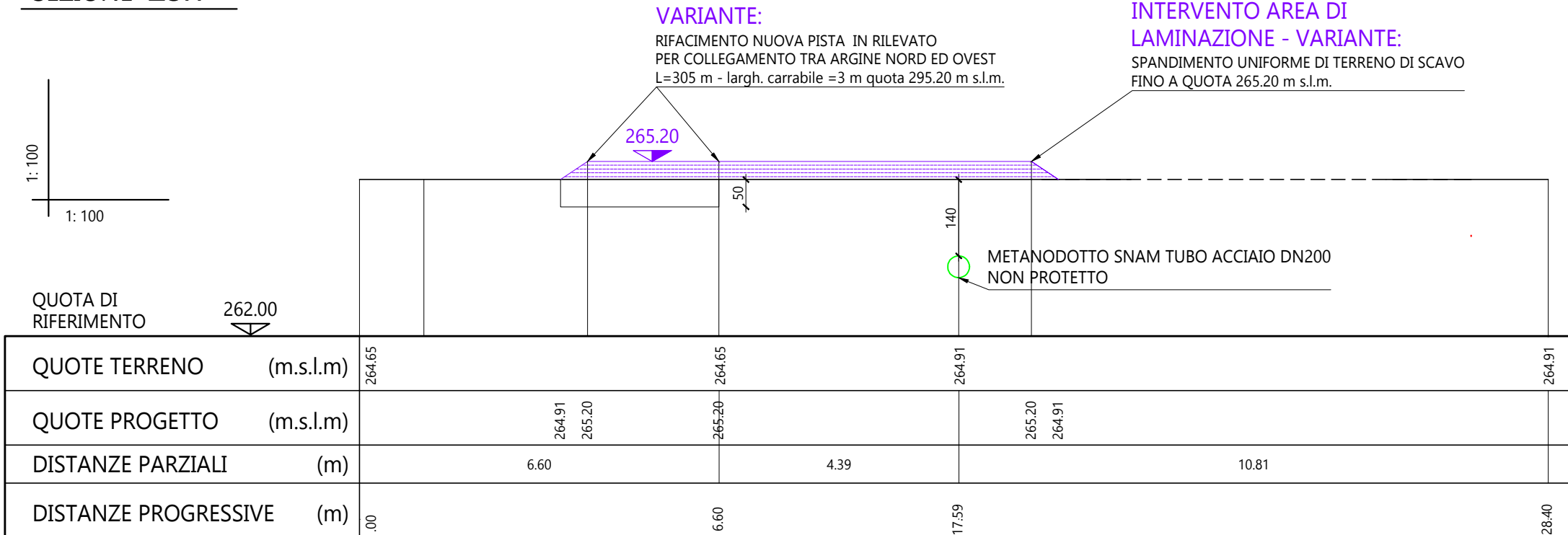
SEZIONE 2 sn
